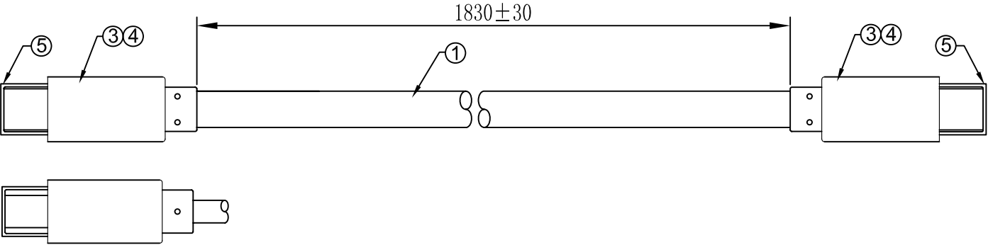
MINI DISPLAYPORT PLUG
