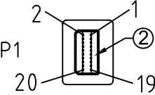
MINI DISPLAYPORT PLUG
