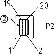
MINI DISPLAYPORT PLUG
